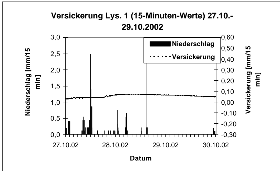
Abb. 6: 15-Minutenwerte des Niederschlags und der Versickerung/Dränspende
