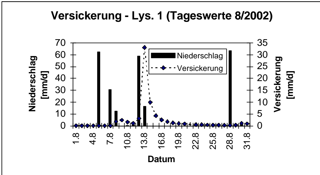
Abb. 3: Tageswerte des Niederschlags und der Versickerung/Dränspende
