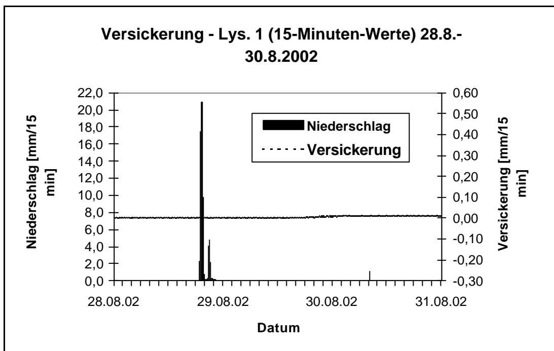
Abb. 4b: 15-Minuten-Werte des Niederschlags und der Versickerung/Dränspende
