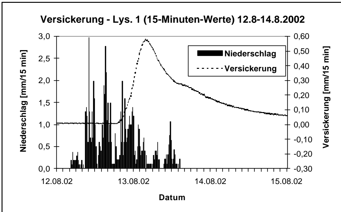
Abb. 4a: 15-Minutenwerte des Niederschlags und der Versickerung/Dränspende
