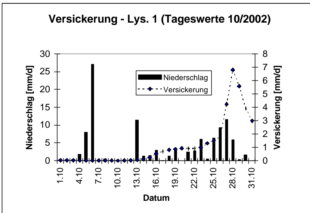
Abb. 5: Tageswerte des Niederschlags und der Versickerung/Dränspende
