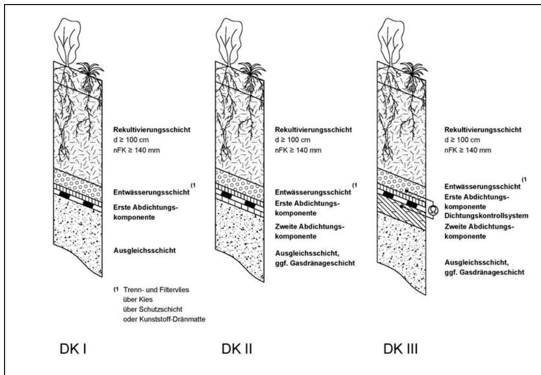
Bild 2: Oberflächenabdichtungssysteme nach DepV (2009)
