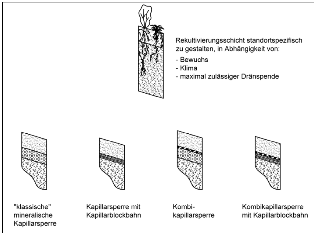
Bild 4: Aufbau unterschiedlicher zulässiger Kapillarsperrensysteme
